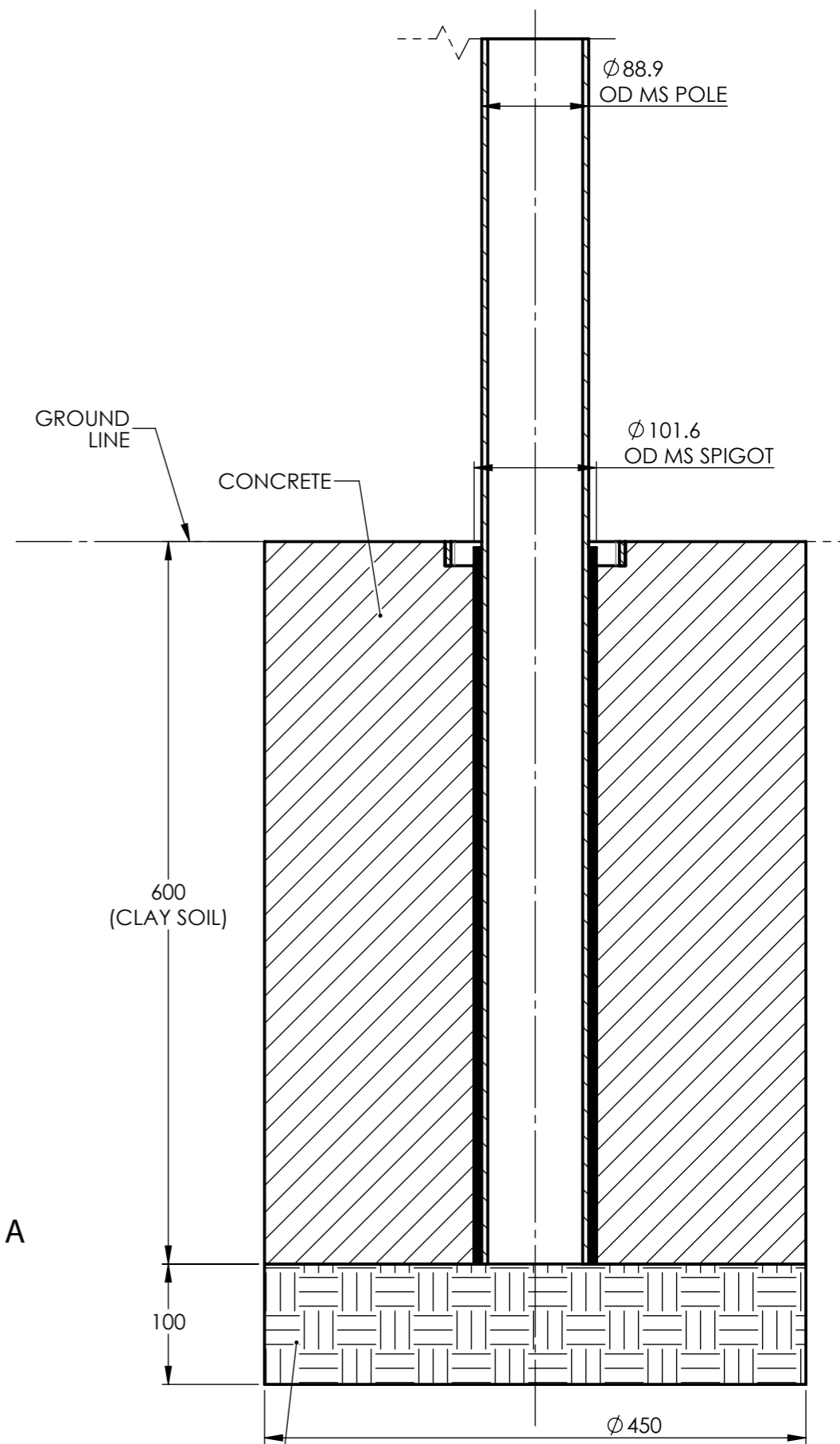
SECTION A-A SCALE 1:5
